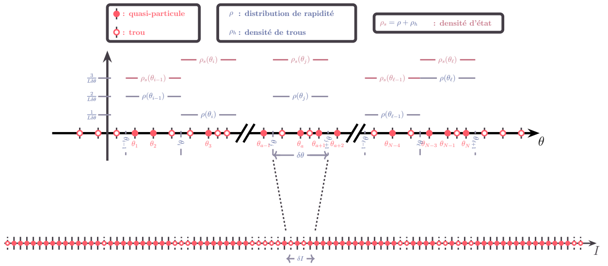
FIGURE I.3 – Illustration de la relation entre la densité d'états \rho_s(\theta) et les nombres quantiques fermioniques I_a . Les rapidités dans l'intervalle [\theta, \theta + \delta\theta] s'associent à un ensemble de nombres quantiques fermioniques situés dans [I, I + \delta I] . La densité d'états \rho_s se déduit alors de la relation \delta I \simeq L\rho_s(\theta)\delta\theta
